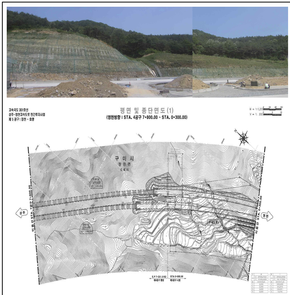
【그림 27.14】 상주절토 27 검토대상 비탈면구간
